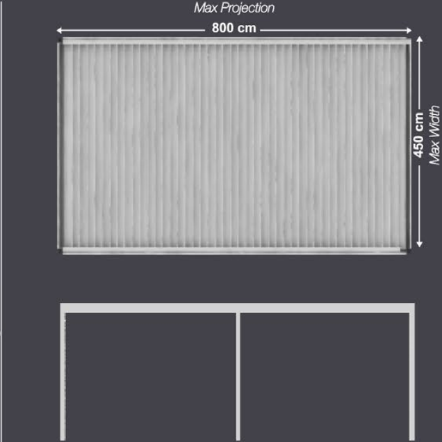
Max. Dimensions
